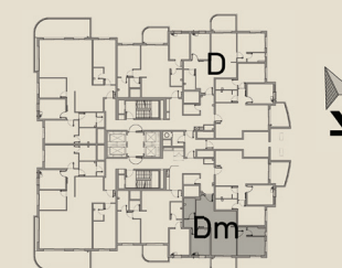
תוכנית קומה 1-9
